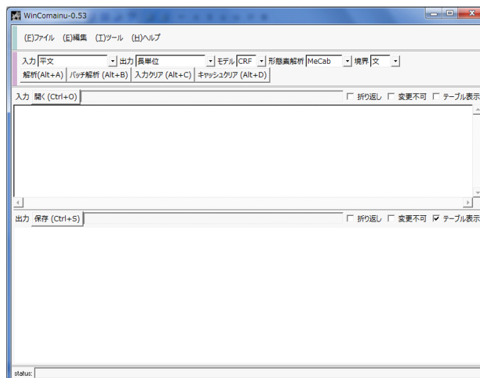
図 2: Comainu(GUI 版)
